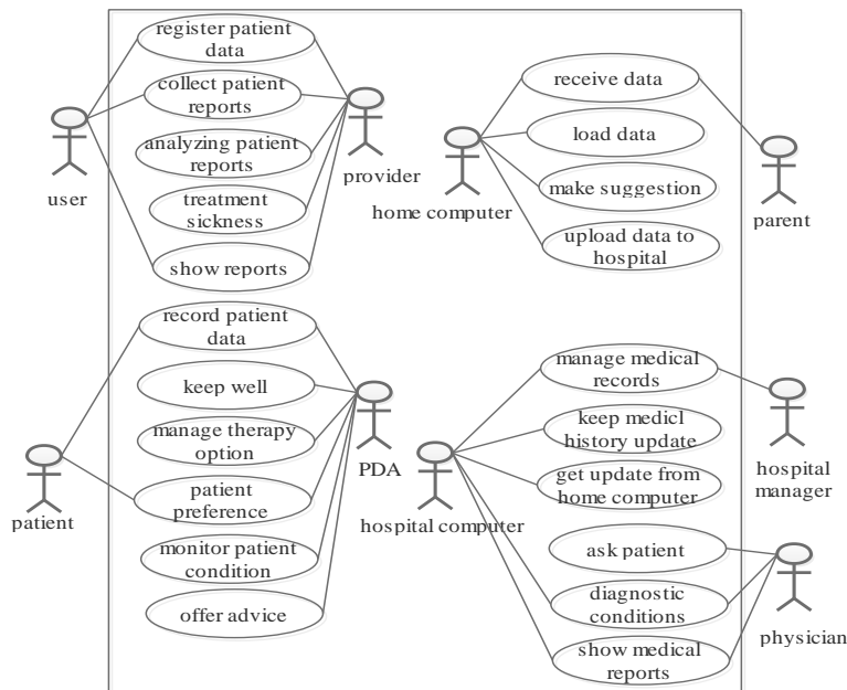
Fig. 7. GA:PCHIS use case diagram
